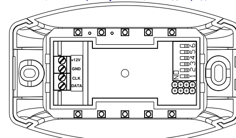
Рисунок 1. ВКП – схема подключения и расположения переключателей.
